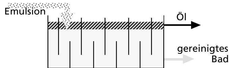
SCHWERKRAFT-ÖLABSCHEIDER
