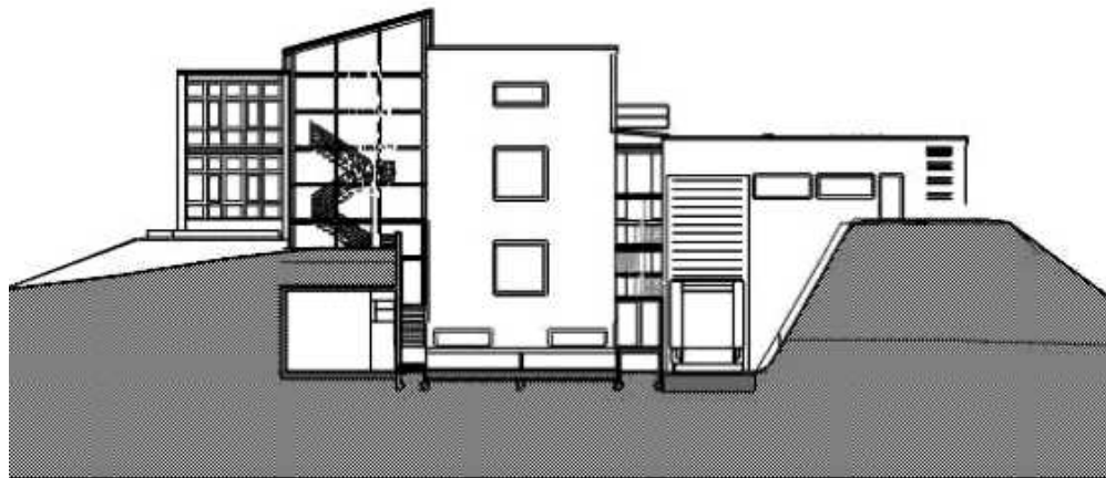
Querschnitt
