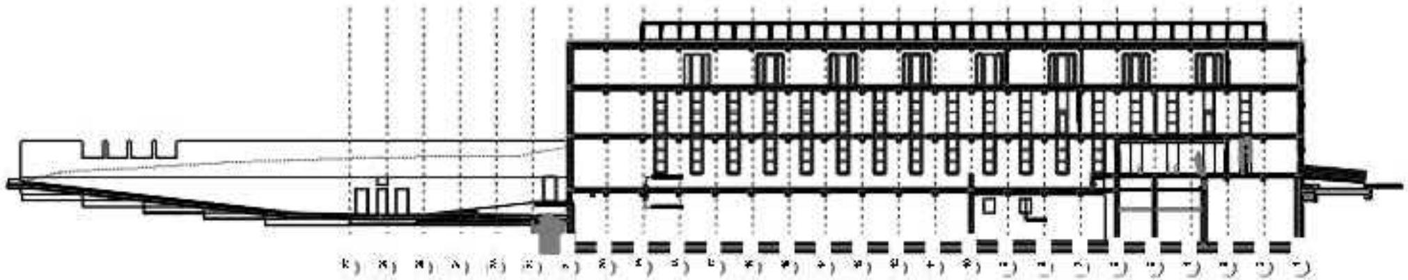
Längsschnitt
